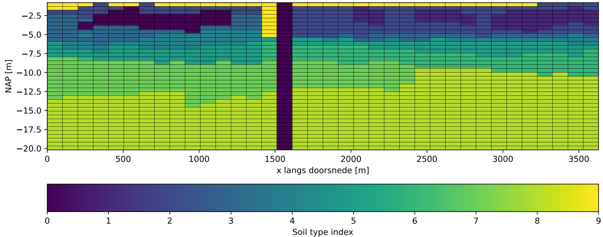
BRO GeoTOP Verticale doorsnede geologische eenheid 128545,477743.pdf with colors converted to soil-indices
